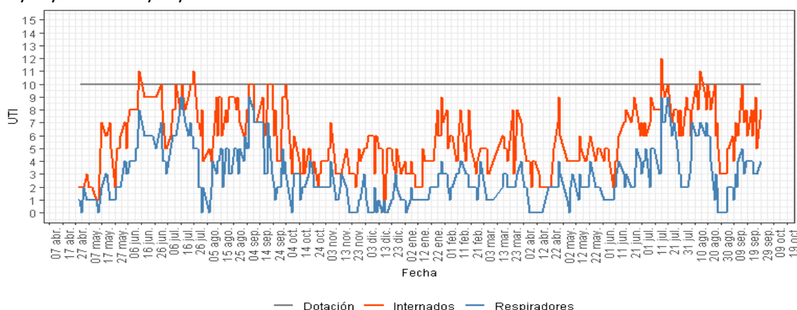
Gráfico 15. Ocupación diaria de las camas de UTI y uso de respiradores. Hospital Vilela, 27/04/2024 a 05/10/2025.
