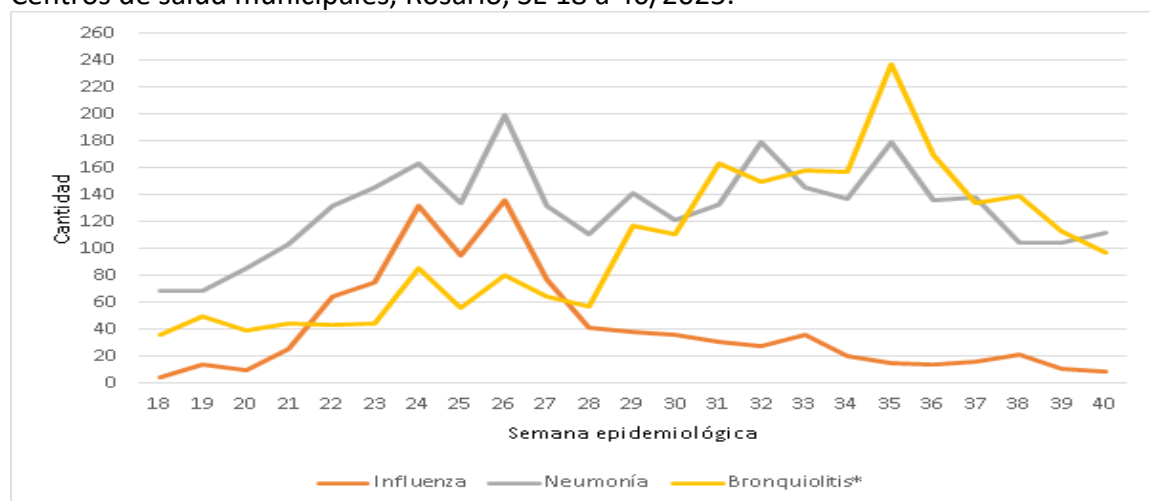
Gráfico 7. Consultas ambulatorias de patología priorizadas según semanas epidemiológicas. Centros de salud municipales, Rosario, SE 18 a 40/2025.
