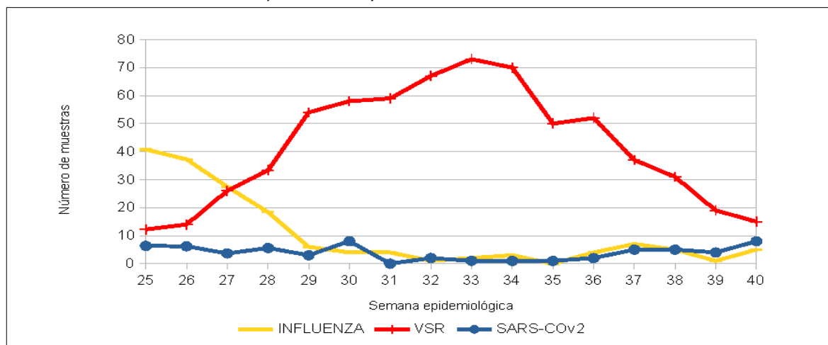
Gráfico 4. Relación de positividad en pacientes testeados para SARS-CoV-2, Influenza y VSR. Laboratorio CEMAR. Rosario, SE 25 a 40/2025.
