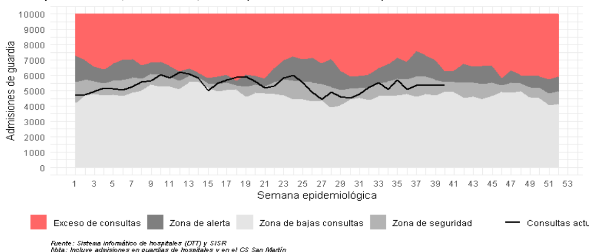
Gráfico 12. Atenciones de guardia y límites de control según semana epidemiológica. Red municipal. Rosario, SE 01 a 40/2025. (frecuencia absoluta)
