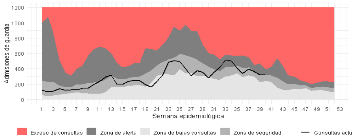
Gráfico 5. Atenciones de guardia por patologías respiratorias y límites de control según semana epidemiológica. Red municipal. Rosario, SE 01 a 40/2025. (frecuencia absoluta)
