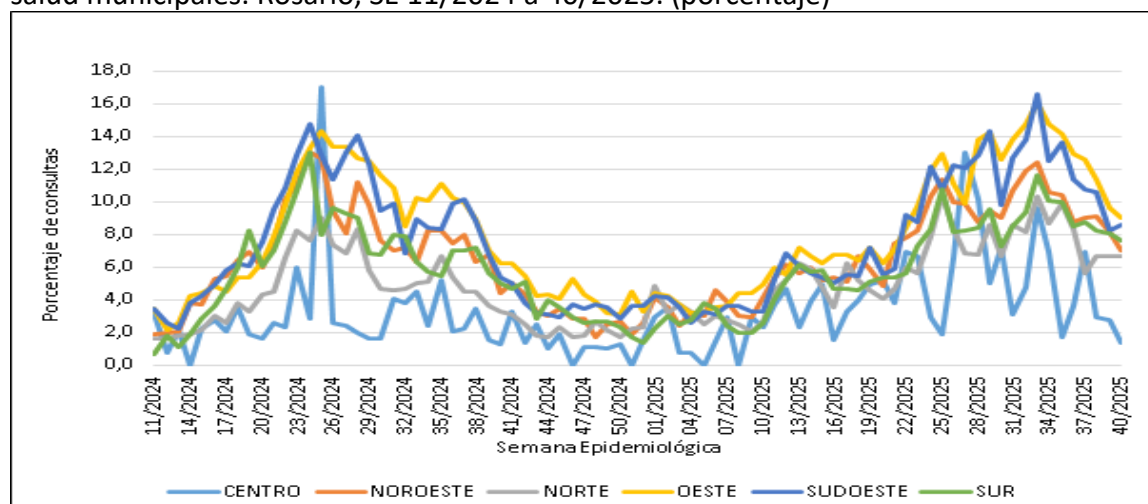
Gráfico 6. Consultas ambulatorias por patologías respiratorias según distrito. Centros de salud municipales. Rosario, SE 11/2024 a 40/2025. (porcentaje)
