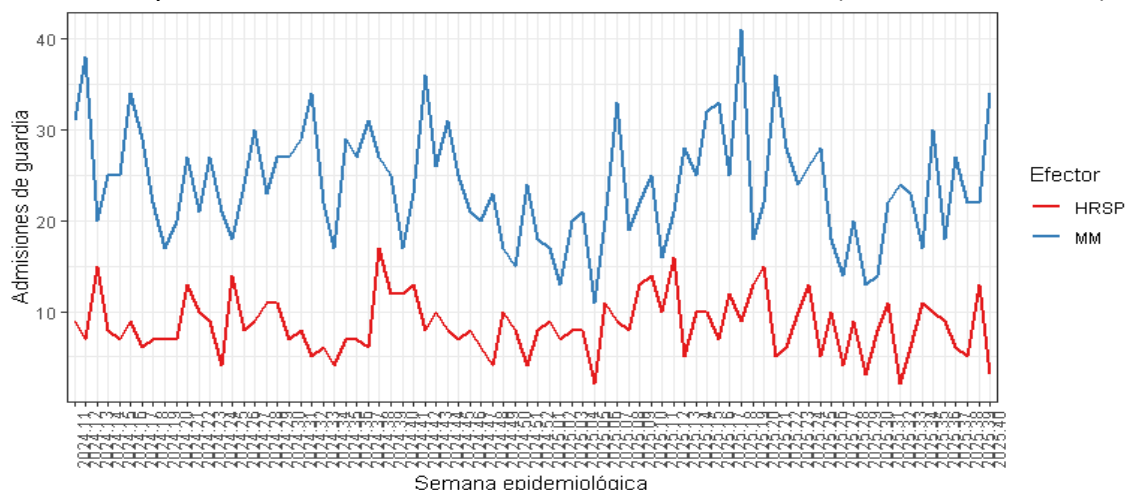
Gráfico 9. Atenciones en guardia neonatológica según semana epidemiológica. Hospital Sáenz Peña y Maternidad Martín. Rosario, SE 11/2024-40/2025. (frecuencia absoluta)
