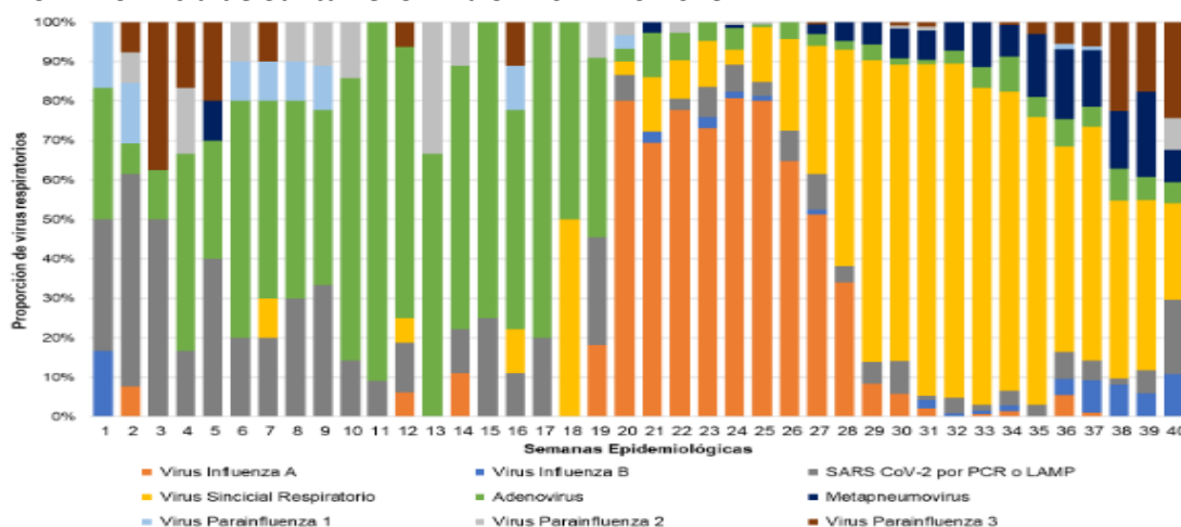
Gráfico 1. Distribución de casos positivos de virus respiratorios en pacientes internados IRA según SE. Provincia de Santa Fe. SE 1 a SE 40 - Año 2025.
