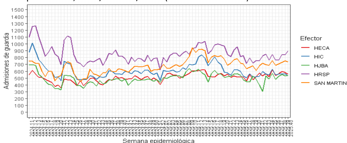
Gráfico 11. Atenciones de guardia de adulto según efector y semana epidemiológica. Red municipal. Rosario, SE 11/2024-40/2025. (frecuencia absoluta)
