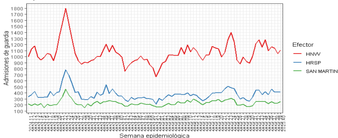
Gráfico 10. Atenciones de guardia pediátrica según semana epidemiológica. Hospitales Vilela, Sáenz Peña y Policlínico San Martín. Rosario, SE 11/2024-40/2025. (frecuencia absoluta)
