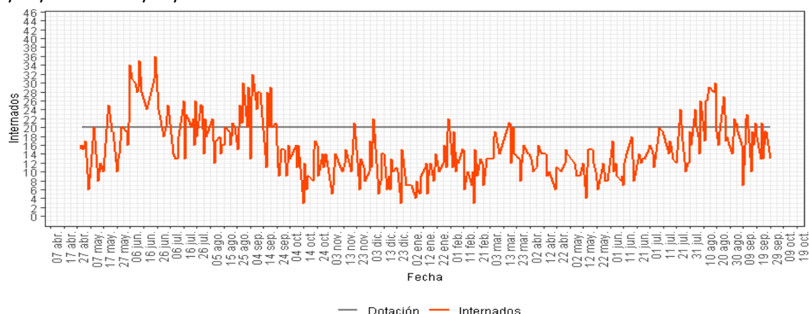
Gráfico 14. Ocupación diaria de camas en internación transitoria del Hospital Vilela. Rosario, 27/04/2024 al 05/10/2025.
