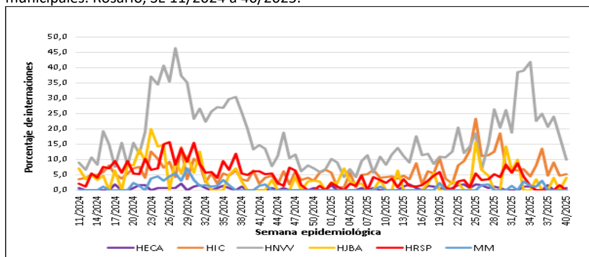
Gráfico 8. Porcentaje de ingresos a internación por patologías respiratorias. Hospitales municipales. Rosario, SE 11/2024 a 40/2025.
