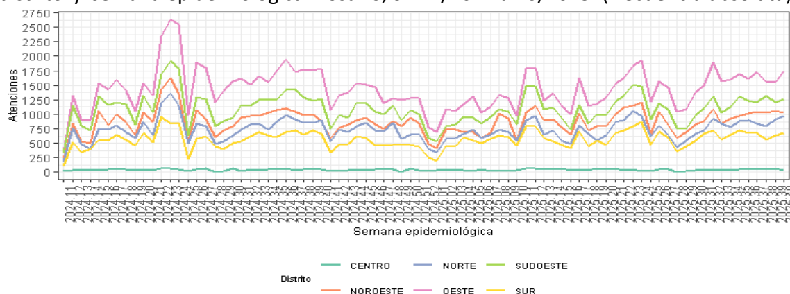
Gráfico 13. Consultas ambulatorias de población infantil en centros de salud según distrito y semana epidemiológica. Rosario, SE 11/2024 a 40/2025. (frecuencia absoluta)
