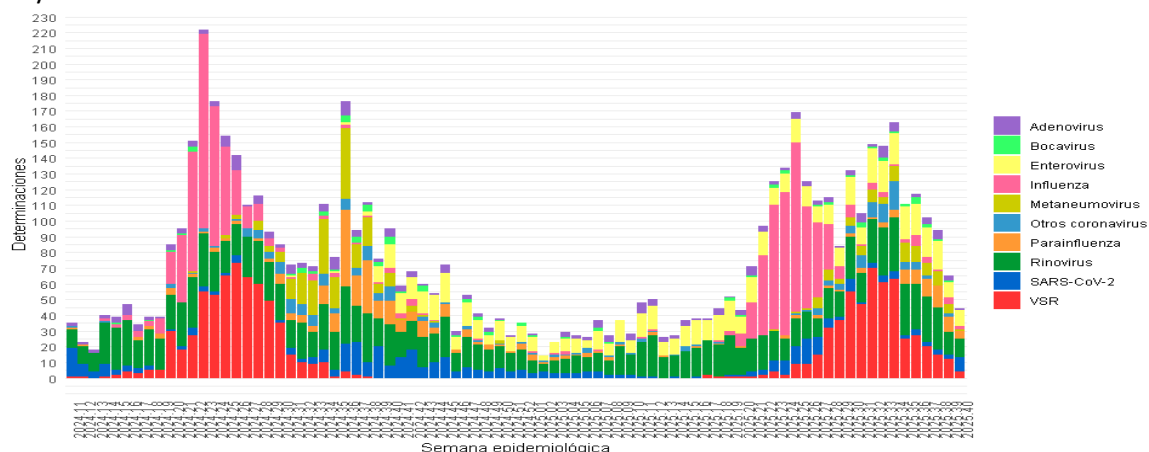
Gráfico 2. Determinaciones positivas de virus respiratorios según virus. Rosario, SE 11/2024 a 40/2025.
