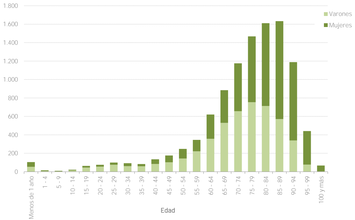
GRÁFICO N°3.2.6: Defunciones de residentes rosarinos registradas en la ciudad de Rosario por sexo y edad. Año 2022
