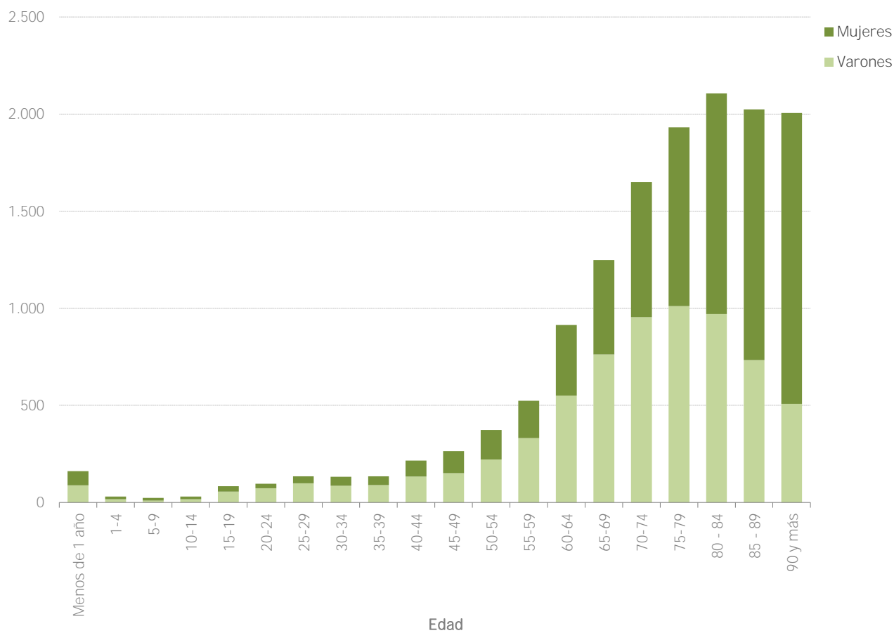
GRÁFICO N°2.6: Defunciones registradas en la ciudad de Rosario por edad y sexo. Año 2022
