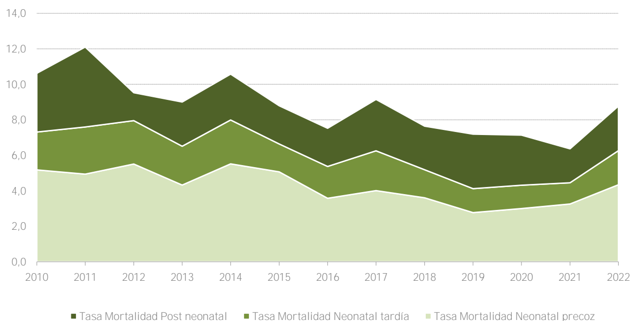
GRÁFICO N°3.3.1: Composición de la tasa de mortalidad infantil, según tiempo de vida de residentes rosarinos. Evolución 2010-2022
