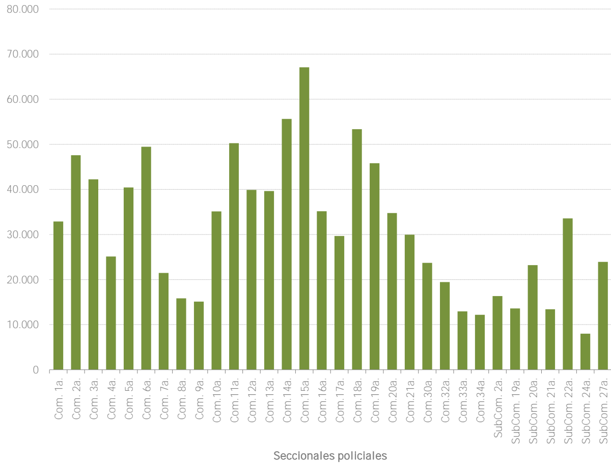
GRÁFICO N°1.2: Población según seccional policial. Año 2022
