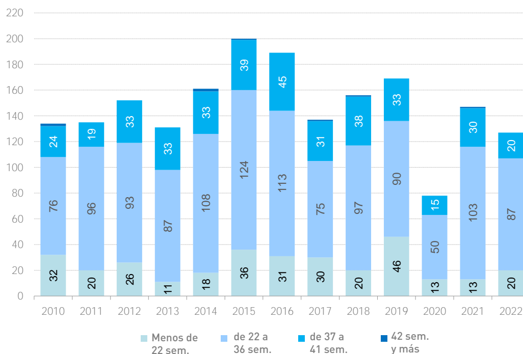
GRÁFICO N°2.10: Defunciones fetales registradas en la ciudad de Rosario por tiempo de gestación (en semanas). Evolución 2010-2022
