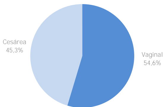
GRÁFICO N°2.3: Nacidos vivos registrados en la ciudad de Rosario por tipo de parto. Año 2022
