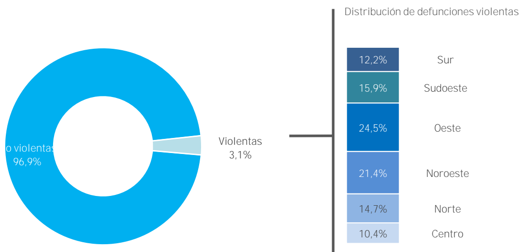
GRÁFICO N°3.2.7: Defunciones de residentes rosarinos registradas en la ciudad de Rosario según tipo de muerte (violenta o no violenta). Año 2022
