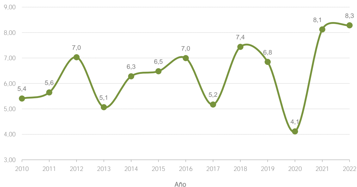
GRÁFICO N°3.4.1: Tasas de mortalidad fetal en la ciudad de Rosario. Evolución 2010 - 2022
