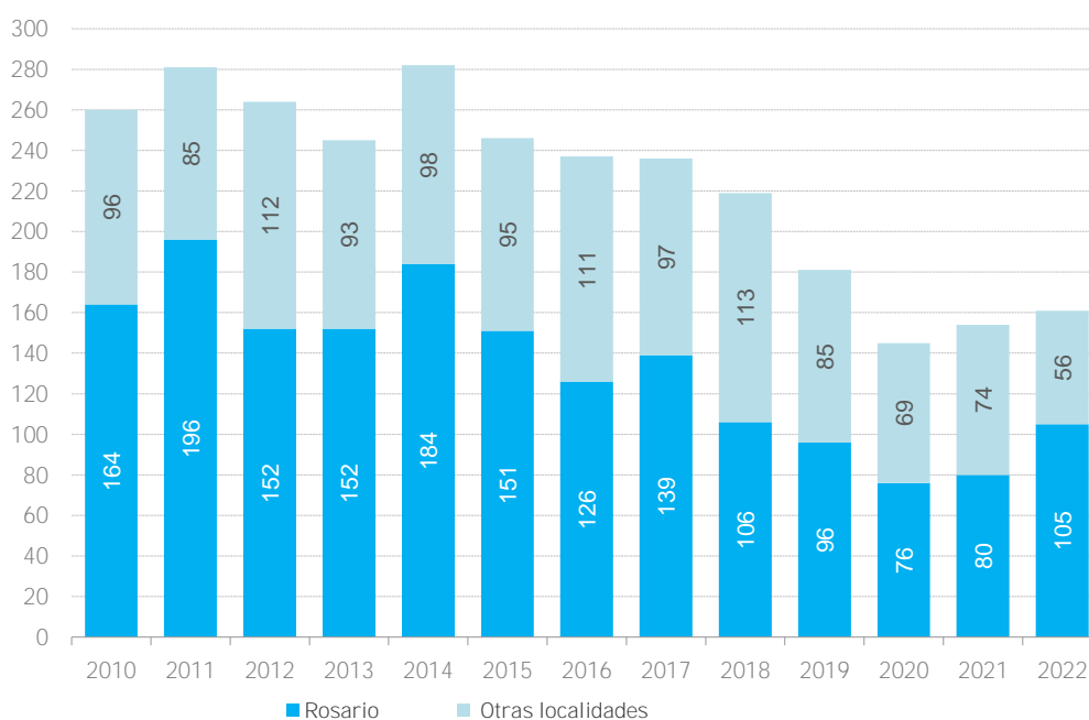
GRÁFICO N°2.7: Defunciones infantiles registradas en la ciudad de Rosario por residencia de la madre. Evolución 2010-2022
