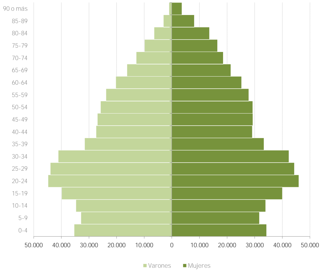
GRÁFICO N°1.1: Pirámide de población de la ciudad de Rosario. Año 2022
