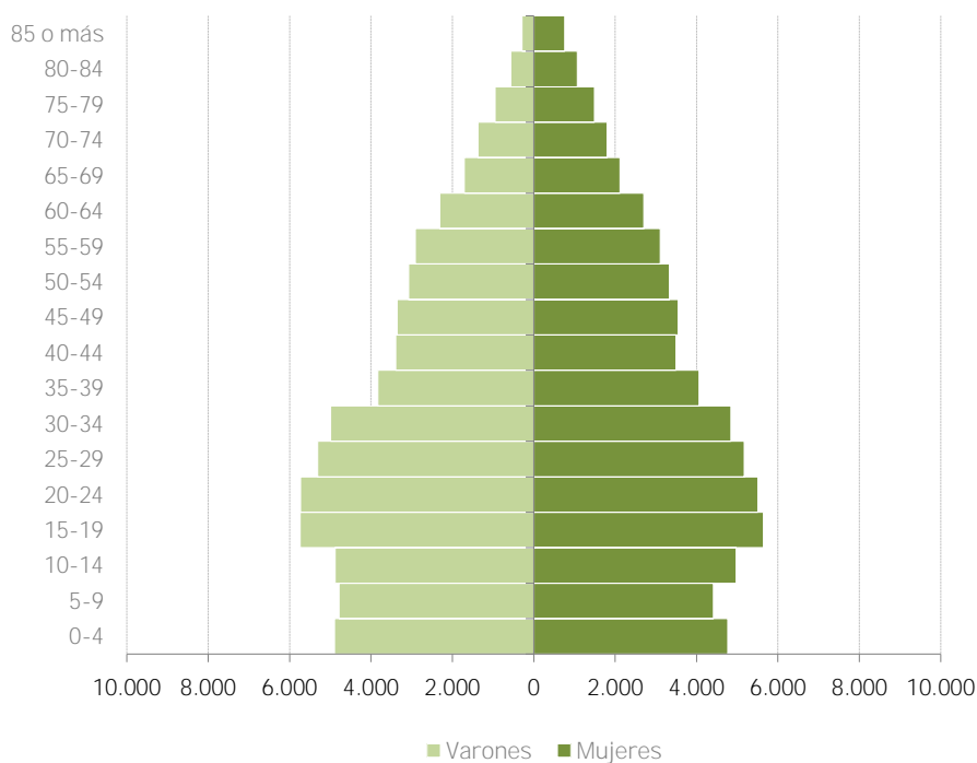
GRÁFICO N°1.6.5: Pirámide de población del distrito Sudoeste. Año 2022
