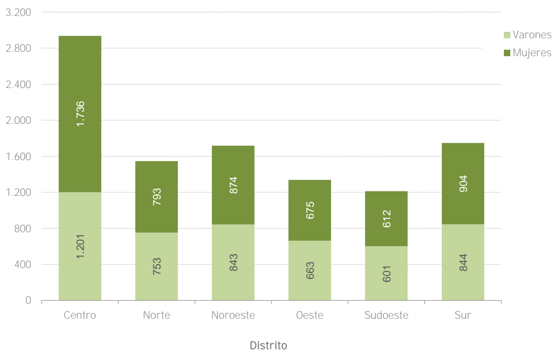
GRÁFICO N°3.2.5: Defunciones de residentes rosarinos registradas en la ciudad de Rosario por sexo y distrito de residencia. Año 2022
