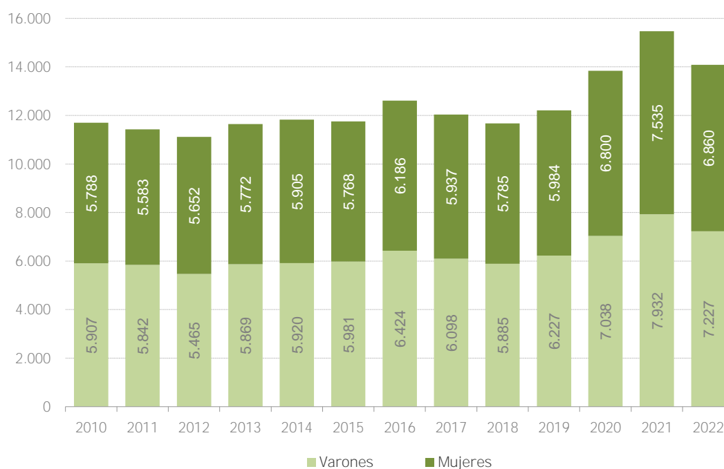
GRÁFICO N°2.5: Defunciones registradas en la ciudad de Rosario por sexo. Evolución 2010-2022
