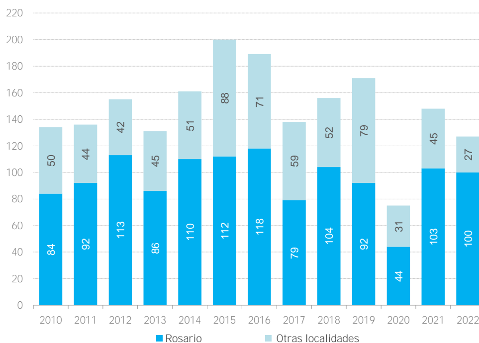
GRÁFICO N°2.9: Defunciones fetales registradas en la ciudad de Rosario por residencia de la madre. Evolución 2010-2022
