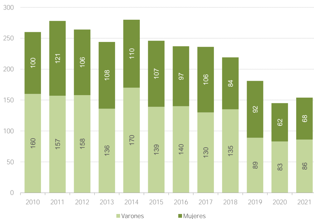
GRÁFICO N°2.8: Defunciones infantiles registradas en la ciudad de Rosario por sexo. Evolución 2010-2022
