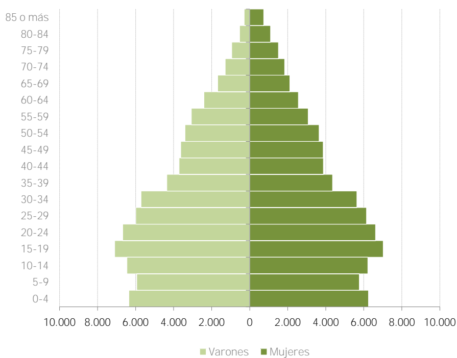
GRÁFICO N°1.6.4: Pirámide de población del distrito Oeste. Año 2022
