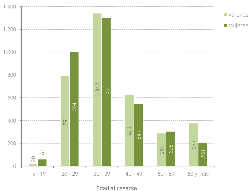
Gráfico N°3.5.3: Contrayentes de matrimonio registrados en la ciudad de Rosario por sexo y edad. Año 2022
