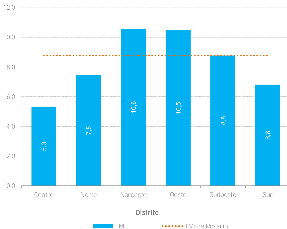
GRÁFICO N°3.3.3: Tasas de mortalidad infantil de residentes rosarinos registradas en la ciudad de Rosario por distrito. Año 2022
