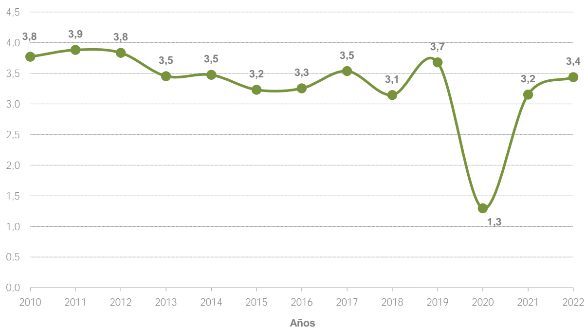
Gráfico Nº3.5.1: Tasas de nupcialidad. Ciudad de Rosario. Evolución 2010-2022
