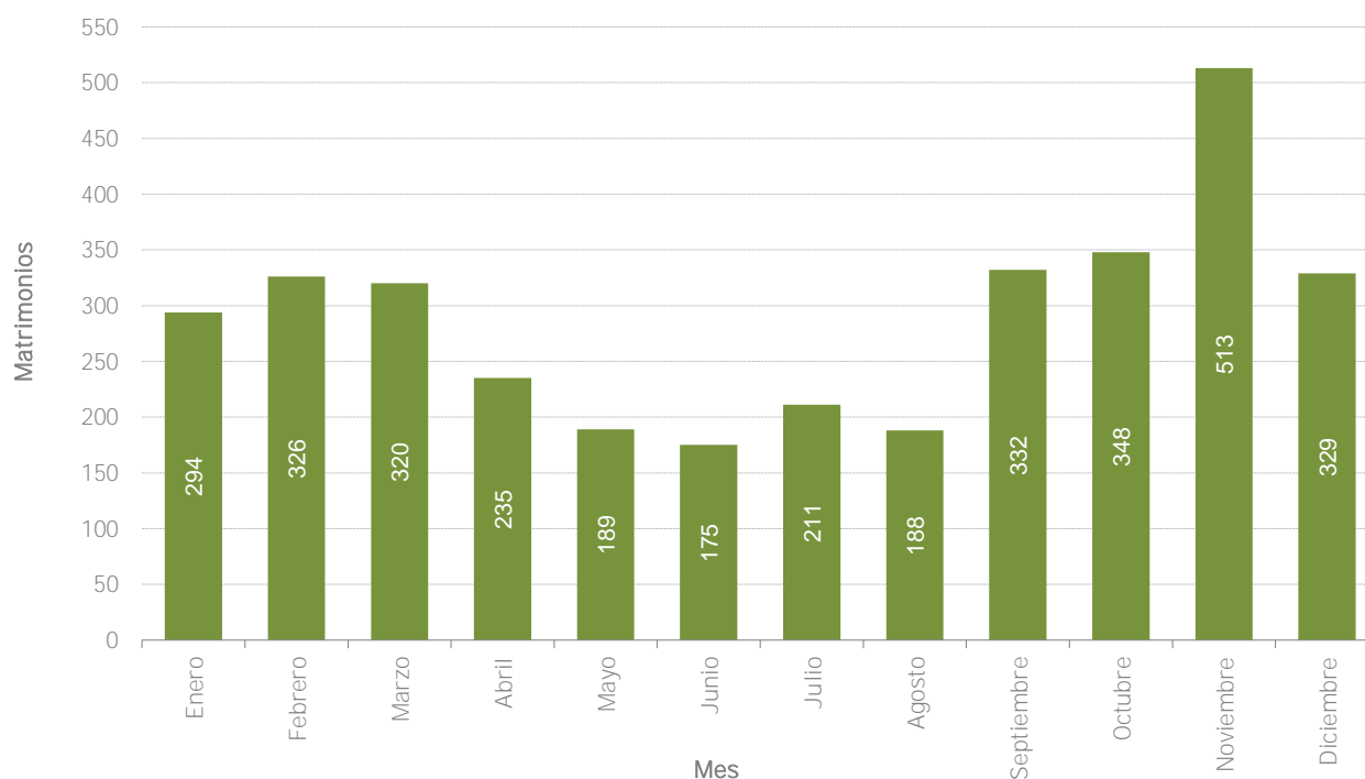
Gráfico N°3.5.2: Matrimonios registrados en la ciudad de Rosario por mes. Año 2022
