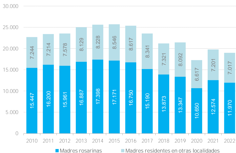
GRÁFICO N°2.1: Nacidos vivos registrados en la ciudad de Rosario por residencia de la madre. Evolución 2010-2022
